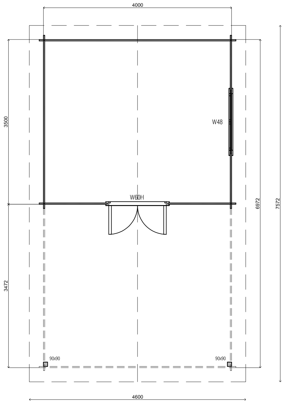
Plattegrond / Plan
