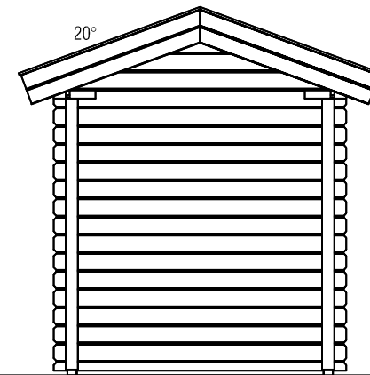
(R) Zijaanzicht / Side view / Seiten ansicht
